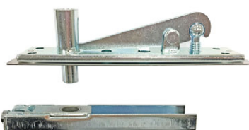
▲ 中心樞軸 200-2P
